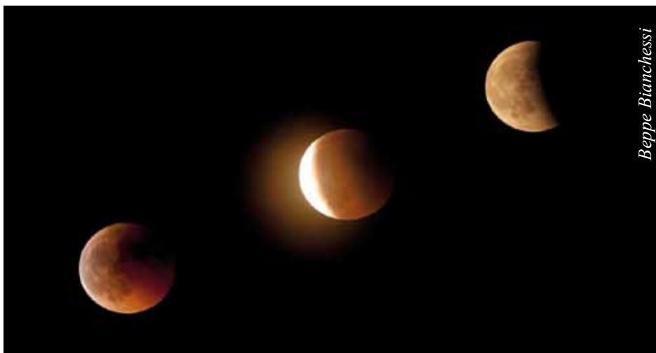
Scatti in sequenza dell'eclissi lunare.
